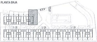
PLANTA BAJA
