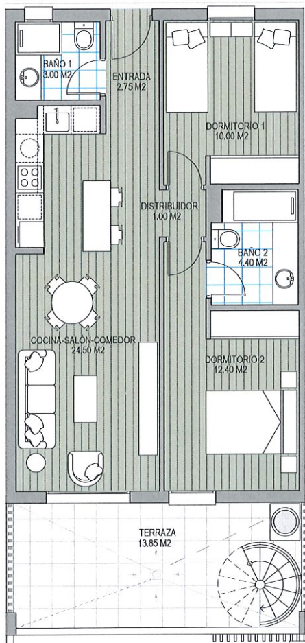
PLANTA ALTA
